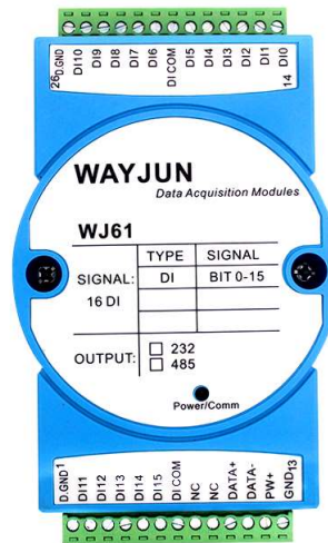
图1 WJ61 模块外观图
